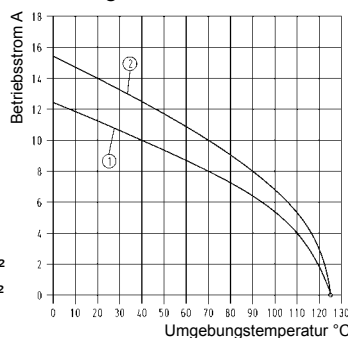
Han D® und Han E® Kontakte mit vergoldeter Oberfläche
