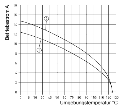
Han D® und Han E® Kontakte mit GoldTec-Oberfläche
