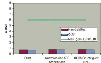
Durchgangswiderstand Gold - GoldTec Han E® Kontakte
