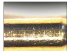
Han E® Kontakte mit GoldTec-Oberfläche nach 500 Steckzyklen
