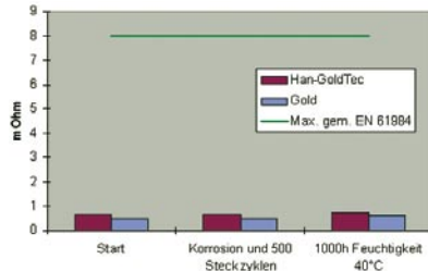
Durchgangswiderstand Gold - GoldTec Han D® Kontakte
